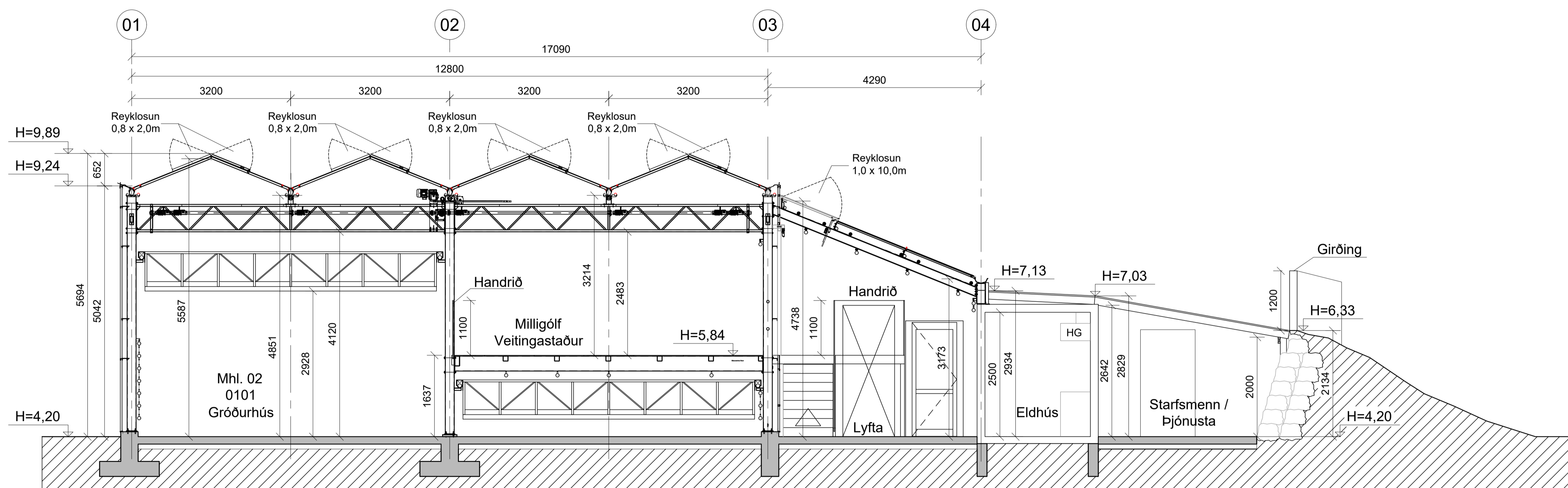
Snið A-A
