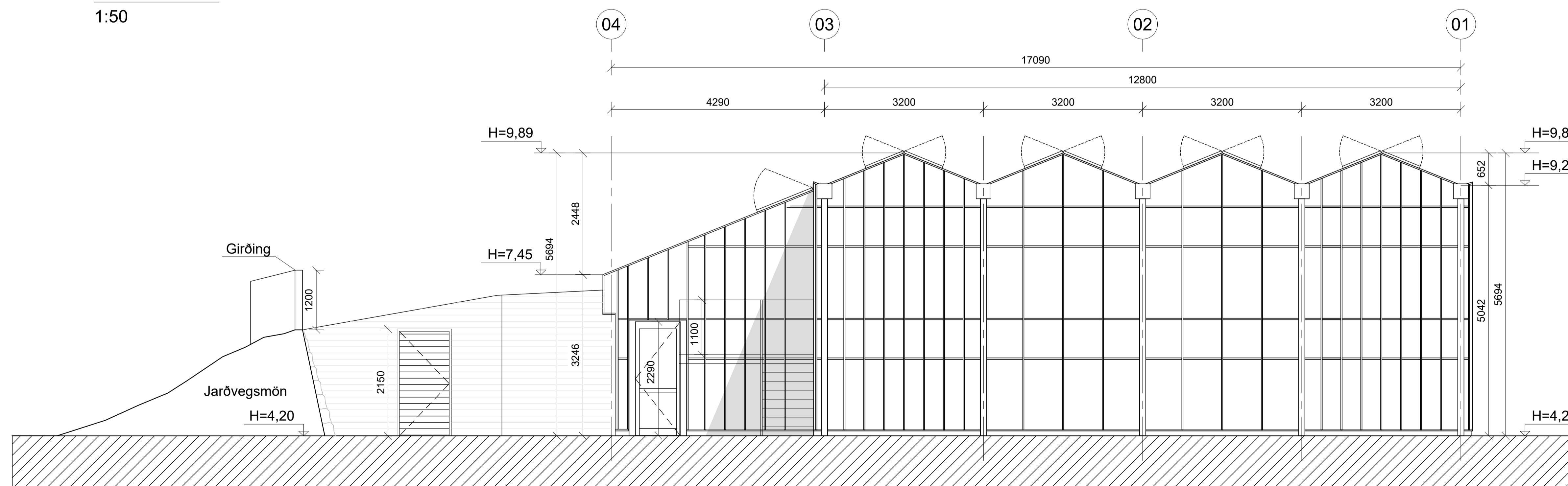
Suður 1:50
